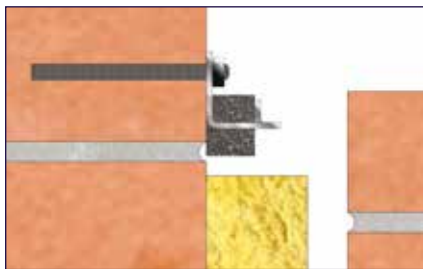
Bevestiging met draadstang M8 + chemische verankering
